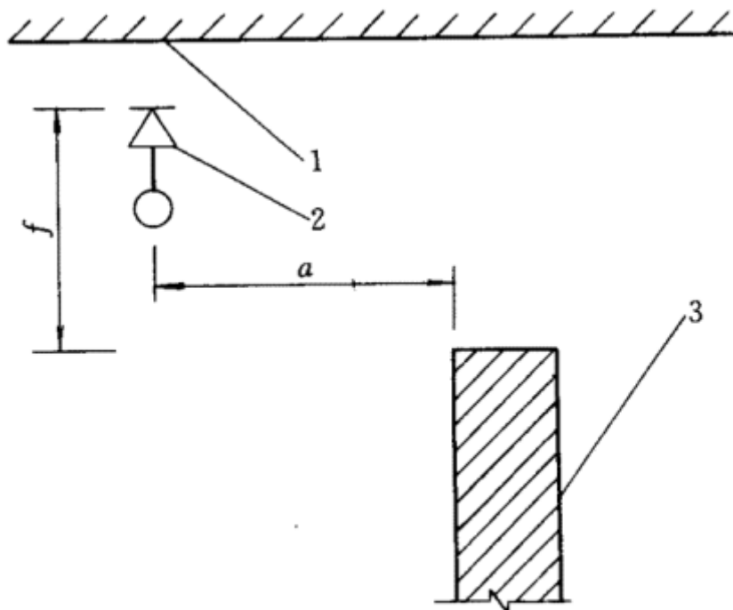
图 7.2.4 喷头与不到顶隔墙的水平距离
