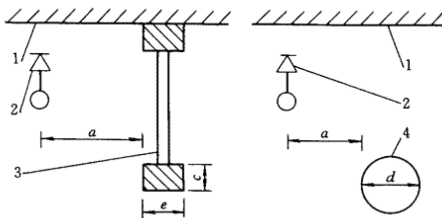
图 7.2.2 喷头与邻近障碍物的最小水平距离
