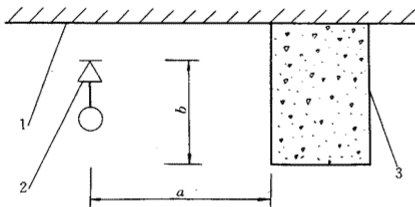
图 7.2.1 喷头与梁、通风管道的距离
