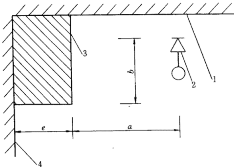
图 7.2.5 喷头与靠墙障碍物的距离
