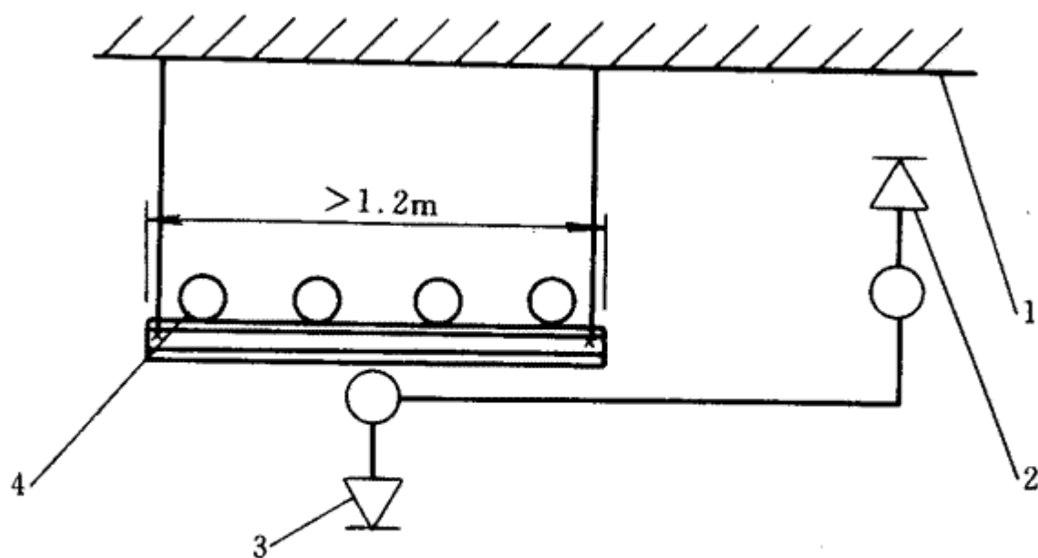
图 7.2.3 障碍物下方增设喷头
